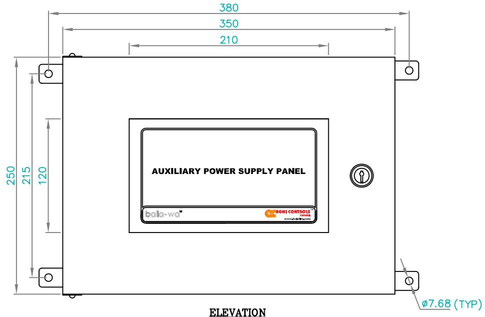
ELEVATION
